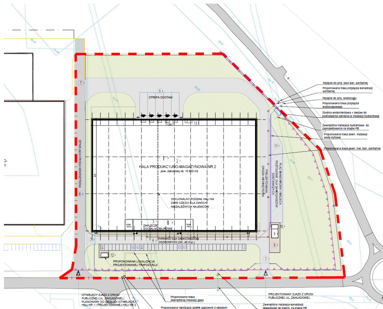
Plan zagospodarowania terenu
