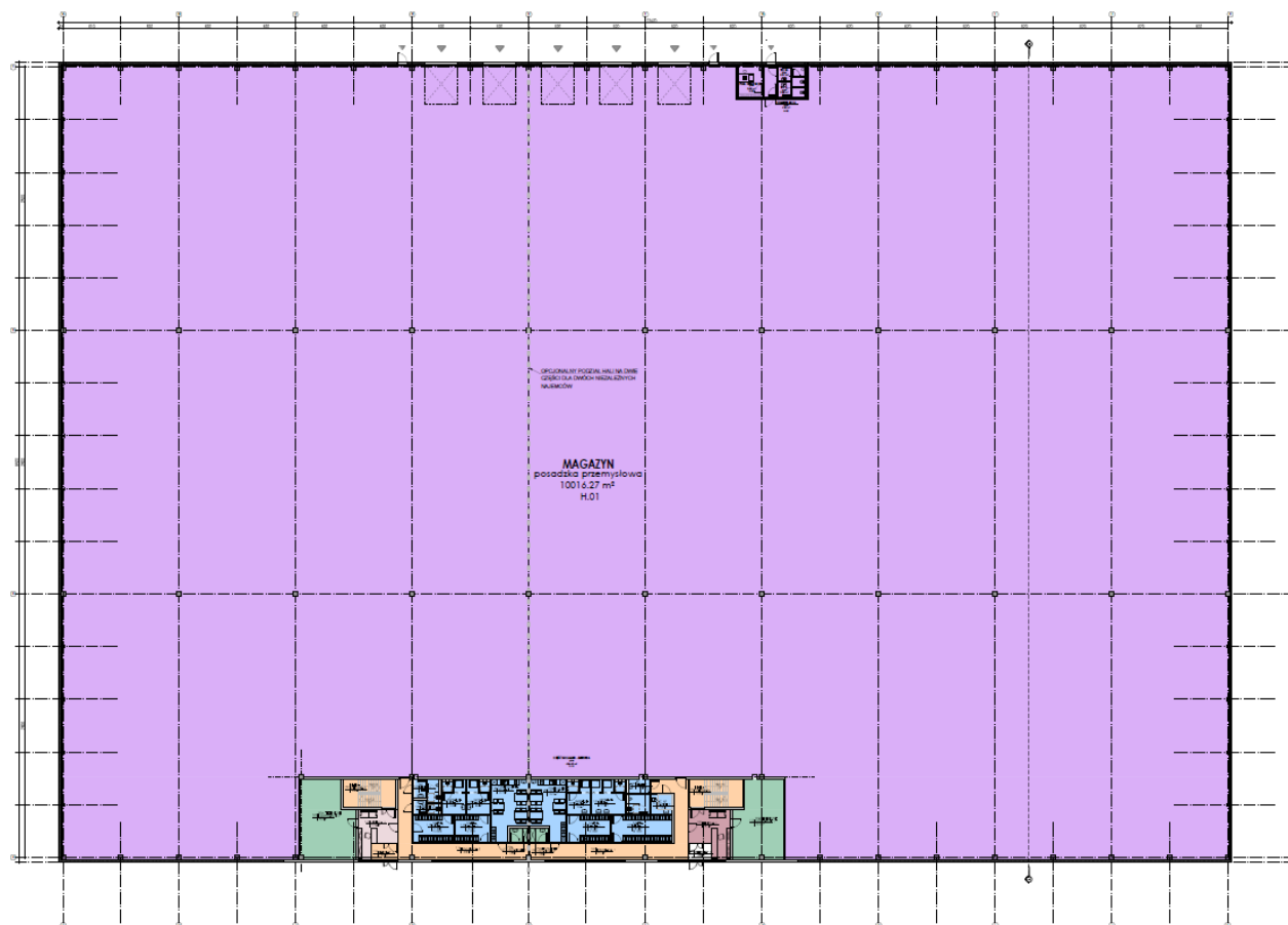
Rzut przyziemia
